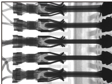
汽车线束
