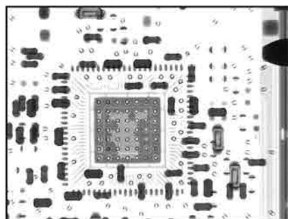
QFN
