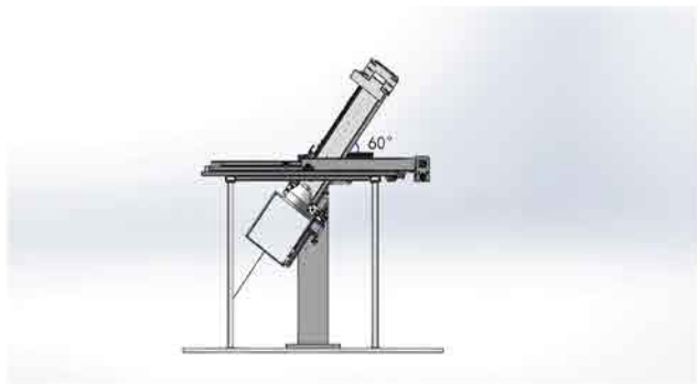
多角度（最大倾斜60°）检测：（不失真变形、不损失能量，不压缩检测范围）
